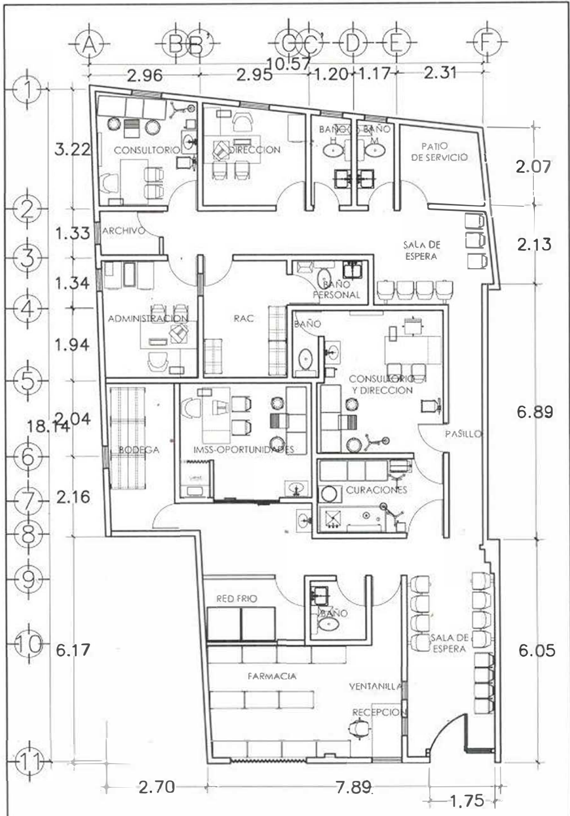
PLANTA ARQ. UMF No.11 UMF NO. 11 ATOYAC DE ALVAREZ, GRO.
