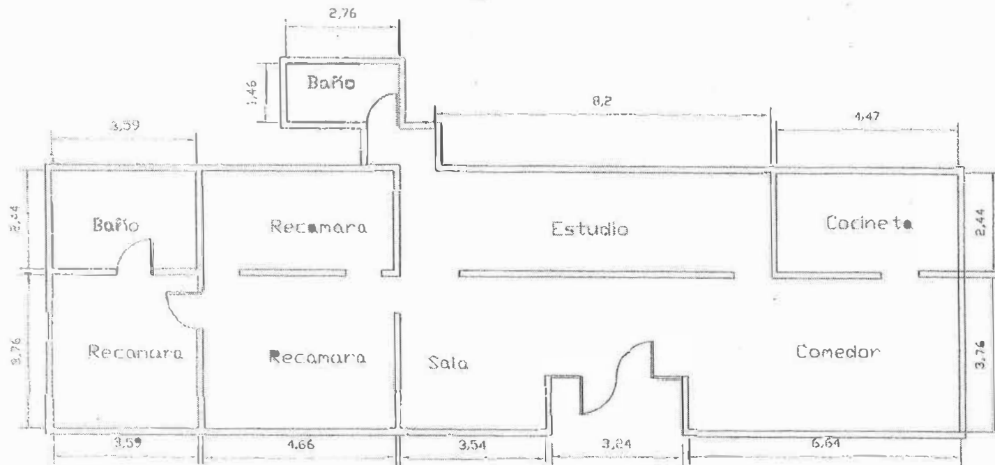
Planta arquitectonica actual
